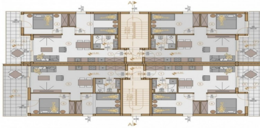
STAMBENE ZGRADE MEDULIN ZGRADA A + B TLOCRT 2. KAT
